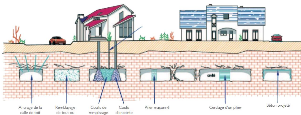
différents types de réduction de l'aléa effondrement de cavité souterraine (source MEED)
